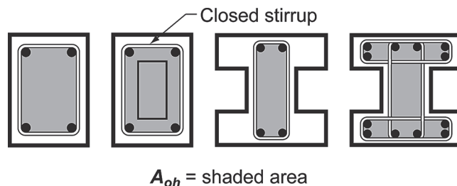
Fig. R22.7.6.1.1—Definition of A_{oh} .
