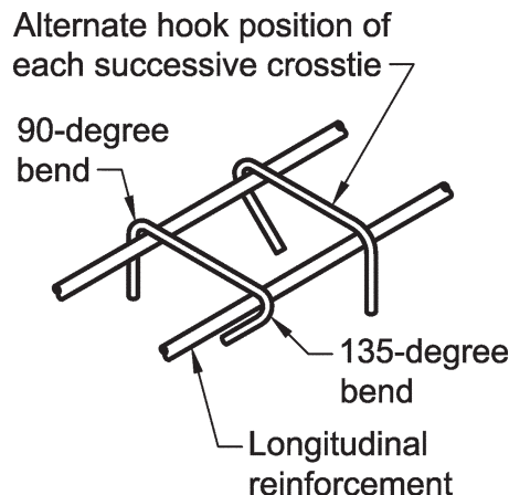
Fig. R25.3.5—Crosstie.
